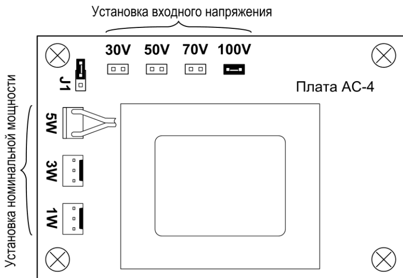
Рис.1 Плата АС
